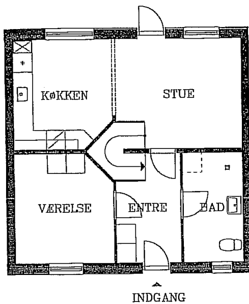
STUEPLAN
